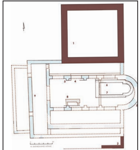
Στο ανώτερο πλάτωμα του ακρωτηρίου, επάνω στα λείψανα του συγκροτήματος του πύργου (με μαύρο) ιδρύθηκε τρίκλιτη παλαιοχριστιανική βασιλική (με γαλάζιο) του 6ου αιώνα. Αποτύπωση: Θ. Μπιλής, Μ. Μαγνήσαλη (αρχιτέκτονες)
