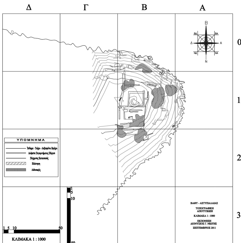
Εἰκ. 1. Τοπογραφικὸ σχέδιο μετὰ τὰ ὁρατὰ λείψανα τῆς θέσης (τοπογράφος: Δ. Νιώτης).
