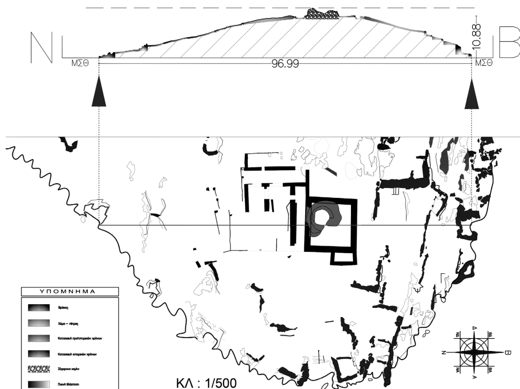
Σχ. 3. Τομή κατά τον άξονα Β.-Ν. του ακρωτηρίου Ἑλληνικό (σχ. Δ. Νιώτης).
