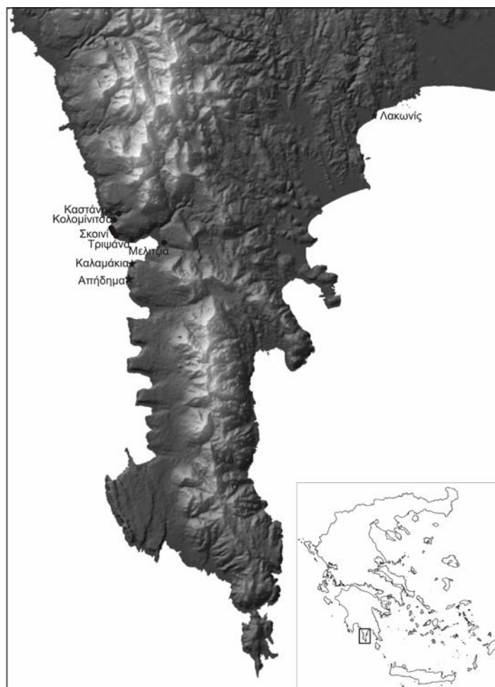
Εικ. 1. Οι ανασκαμμένες παλαιολιθικές θέσεις της Μάνης (με αστερίσκο σημειώνονται οι θέσεις της Μέσης Παλαιολιθικής, με κύκλο εκείνες της Ανώτερης Παλαιολιθικής) (Α. Ντάρλας).
