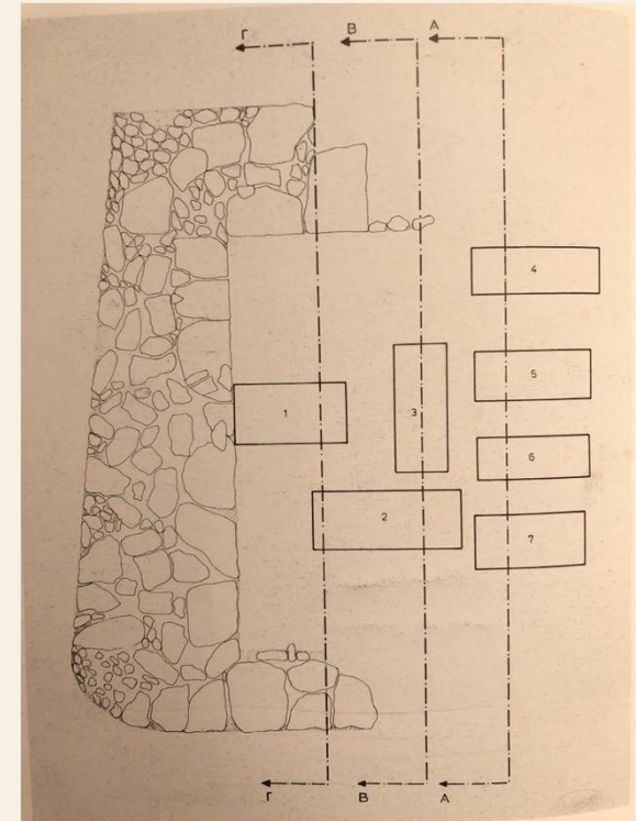
ΕΙΚ. 11: ΚΑΤΟΨΗ ΘΕΣΗΣ ΕΠΙΤΥΜΒΙΩΝ ΣΤΗΛΩΝ
