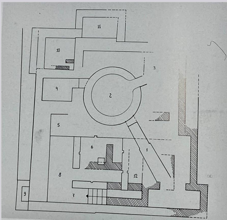
ΕΙΚ.28: ΚΑΤΟΨΗ ΣΥΓΚΡΟΤΗΜΑΤΟΣ ΘΟΛΩΤΟΥ ΤΑΦΟΥ Β
